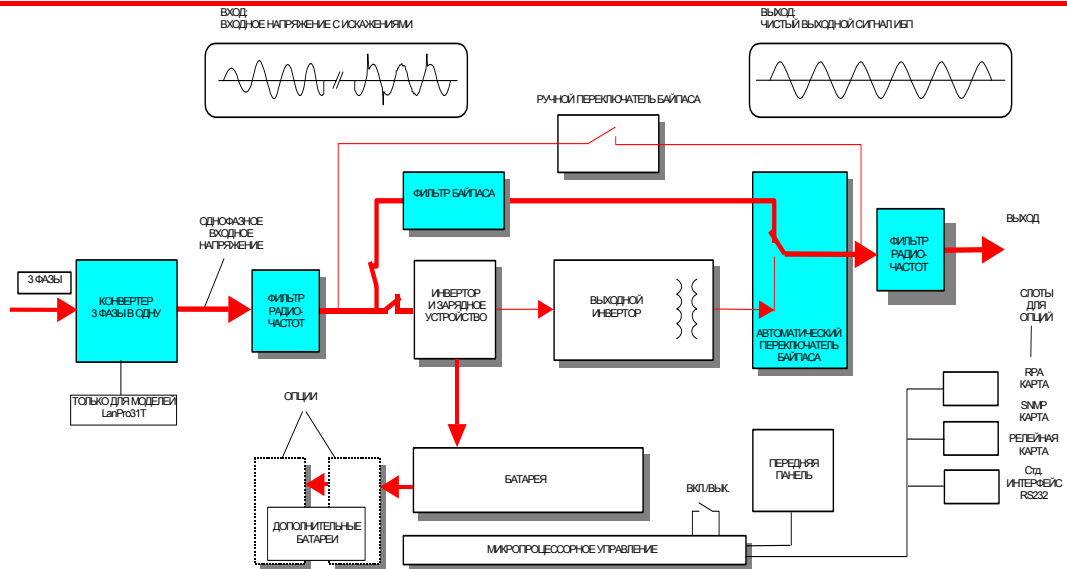
Рис. 3. Схема ИБП LP-11, перебои электропитания.
