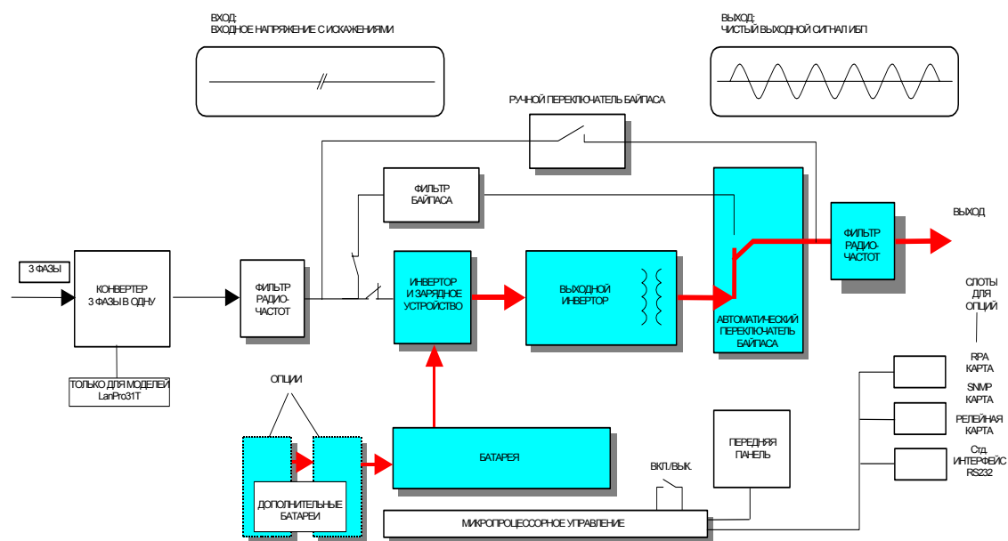
Рис. 2. Блок-схема ИБП LP-11 , электросеть присутствует.
