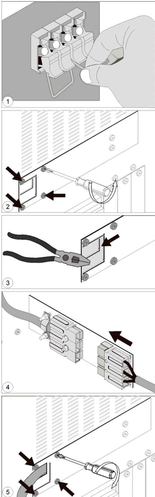
Рис. 7. LP 3/5/6-11: Установка дополнительных батарейных блоков.
