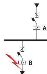
Селективность между T2160 PR221 In100 и S280 C50
