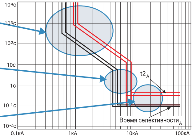
Селективность между Emax
