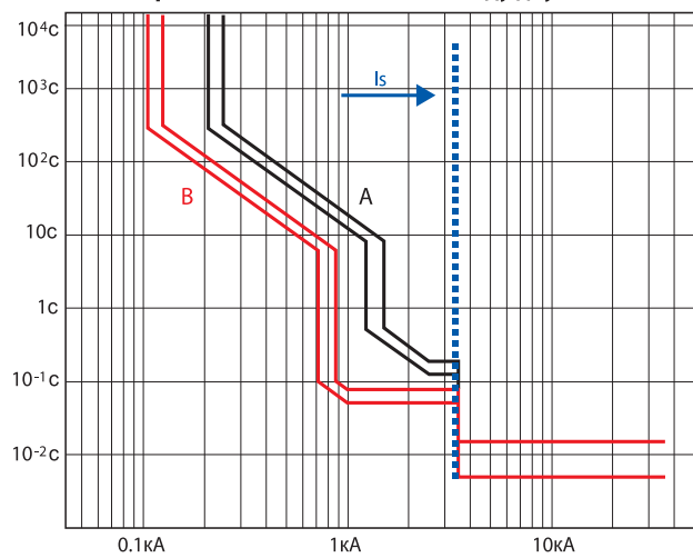
Временная селективность между двумя T4
