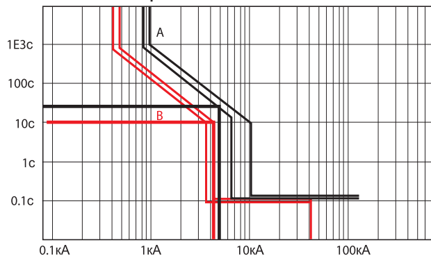
Времятоковая селективность
