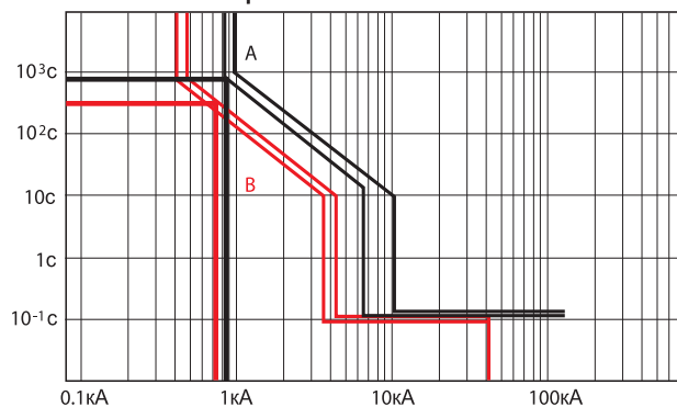
Времятоковая селективность
