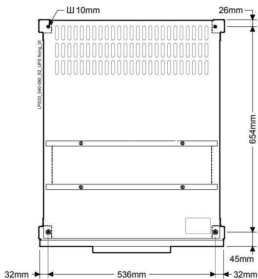
Рис. 5.4-5 LP 33 Series 60 - 80 кВА - UPS - места крепления шкафа ИБП к полу
