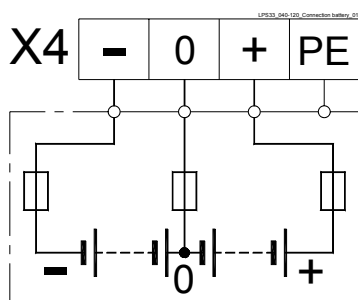
Рис. 5.8.2-2 Подключение внешней батареи
