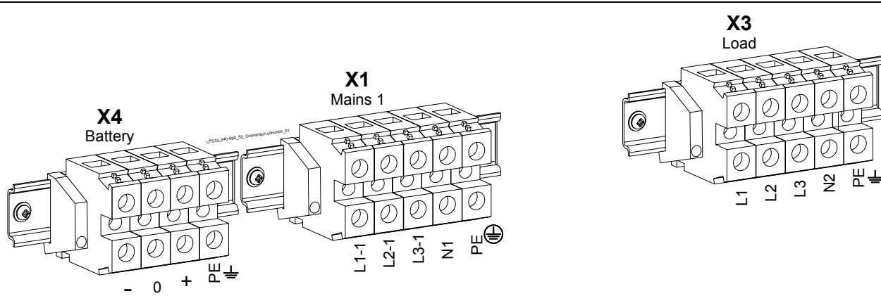
Рис. 5.8.1-1 Клеммы общего входа для подключения к электросети
