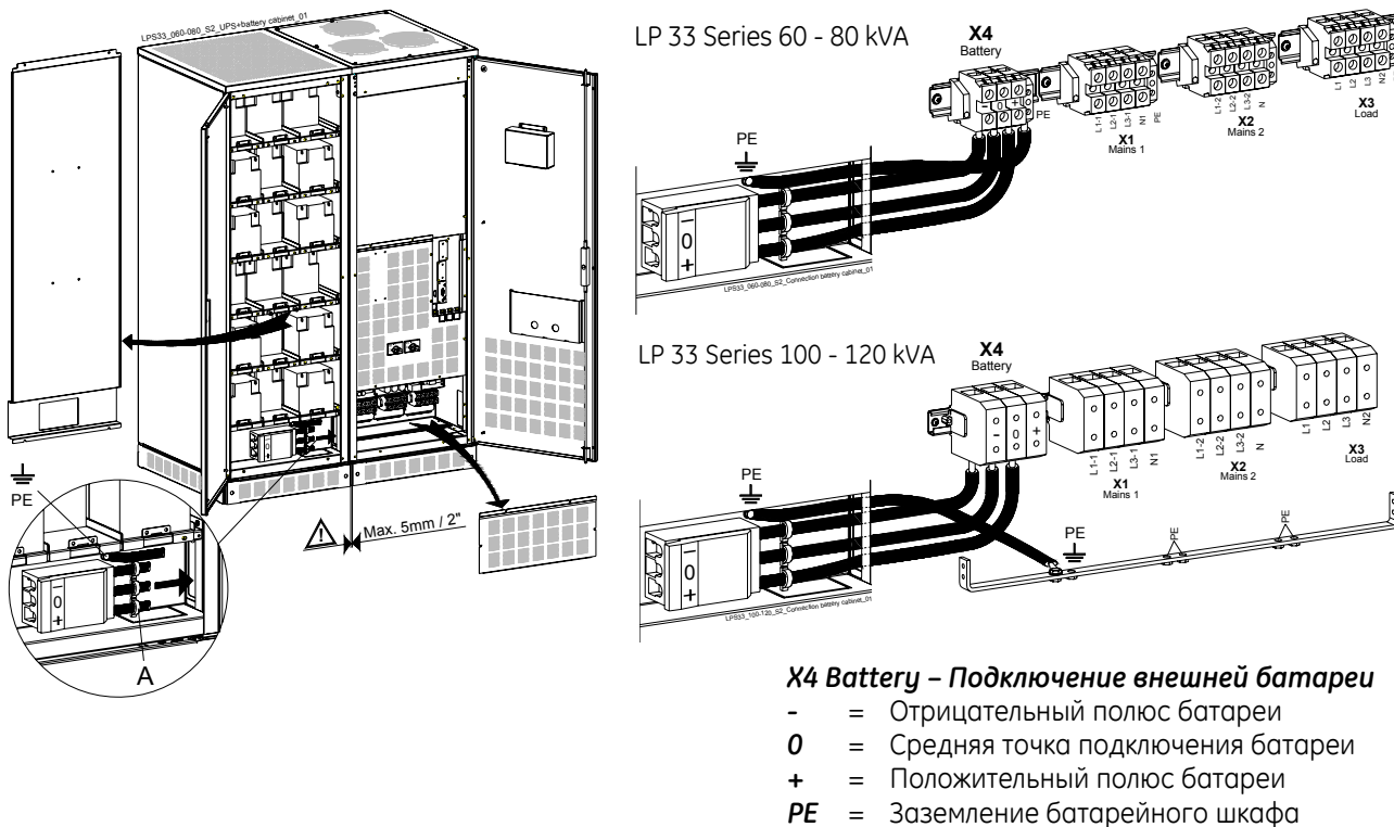
Рис. 10.2.2-1 Расположение и подключение дополнительных батарей
