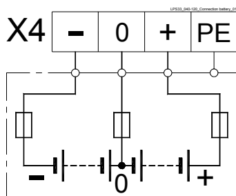
Рис. 5.8.1-2 Подключение внешней батареи
