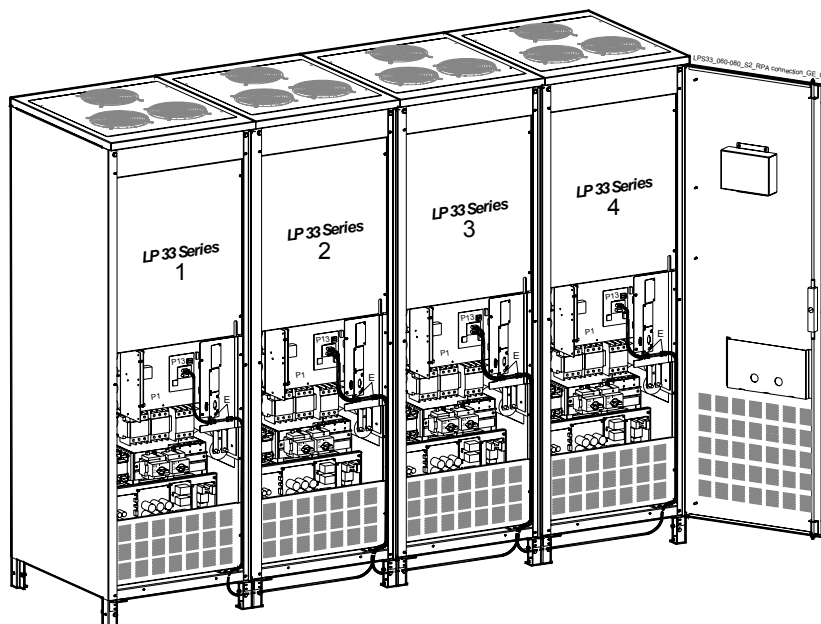
Рис. 5.8.7-5 LP 33 Series 60 - 80 кВА – Расположение шины управления параллельной системой RPA
