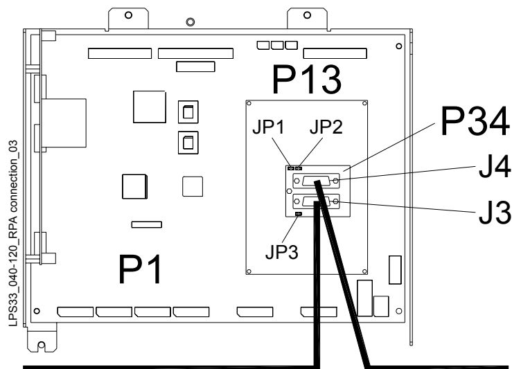
Рис. 5.8.7-4 Подключение к плате «P34 – Connector adapter RPA»
