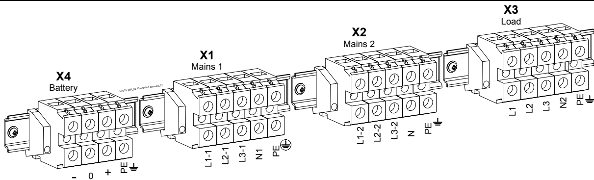
Рис. 5.8.4-1 Клеммы отдельного входа для подключения к электросети
