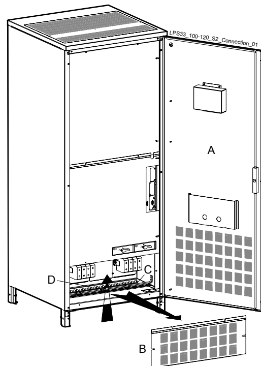
Рис. 5.8-2 LP 33 Series 100 - 120 кВА Подключение силовых кабелей
