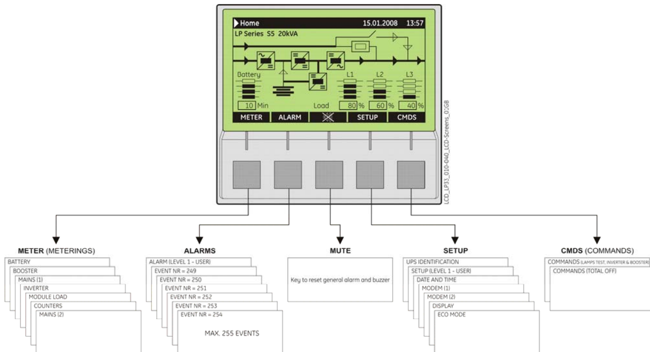
Рис. 7.1-1 ЖК-дисплей
