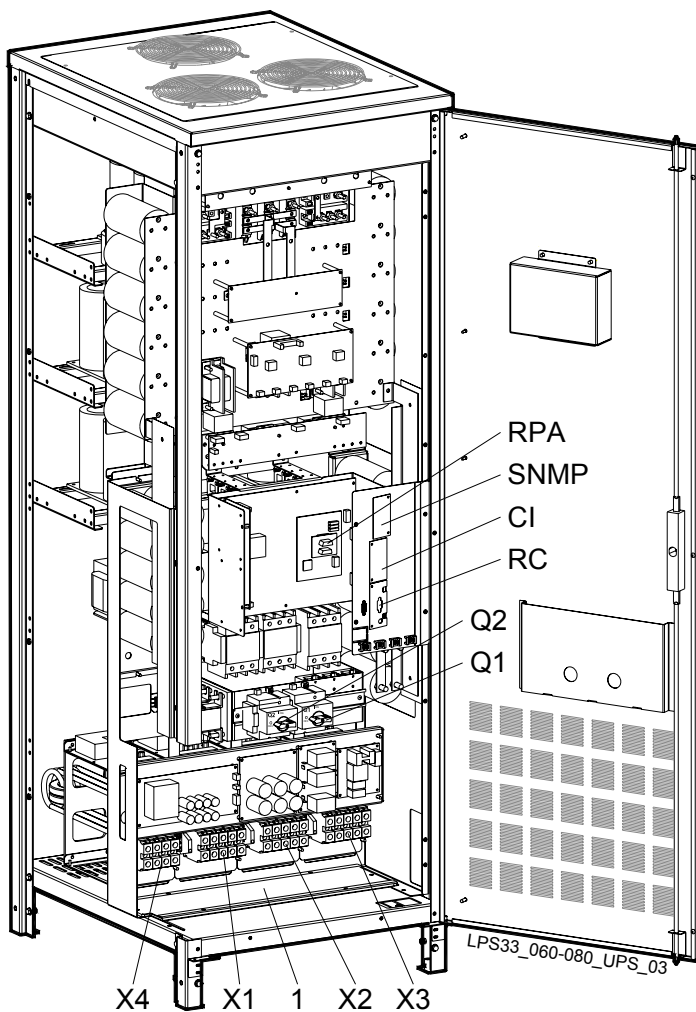
Рис. 2.1-3 Общий вид со снятыми защитными панелями
