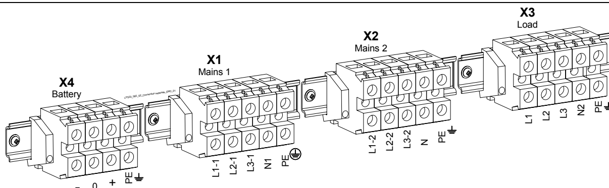
Рис. 5.8.5-1 Клеммы отдельного входа для подключения к электросети
