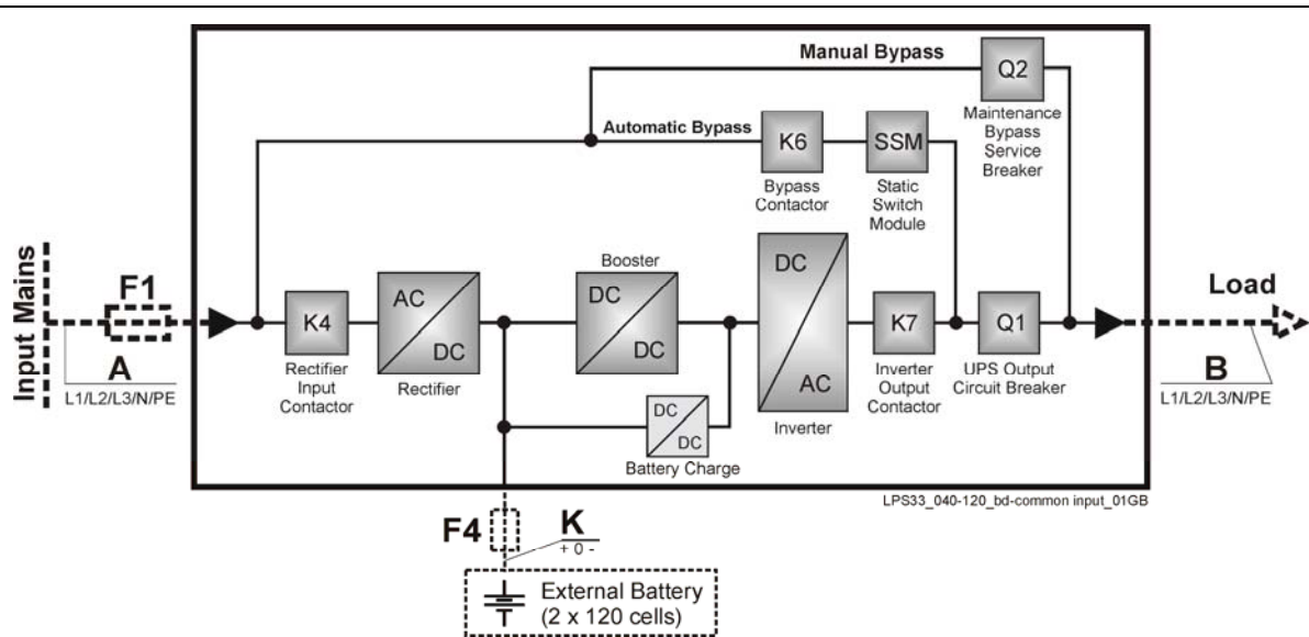
Рис. 5.8-3 Общее подключение электросети
