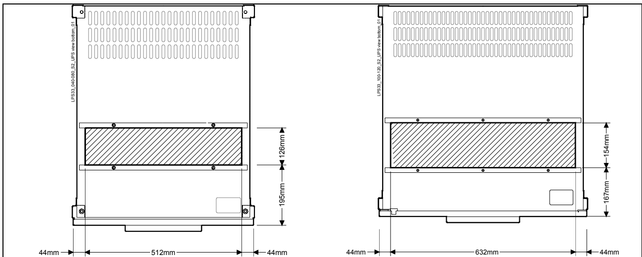
Рис. 5.4-2 LP 33 Series 60 - 80 кВА - Отверстие на нижней панели шкафа Рис. 5.4-3 LP 33 Series 100 - 120 кВА - Отверстие на нижней панели шкафа
