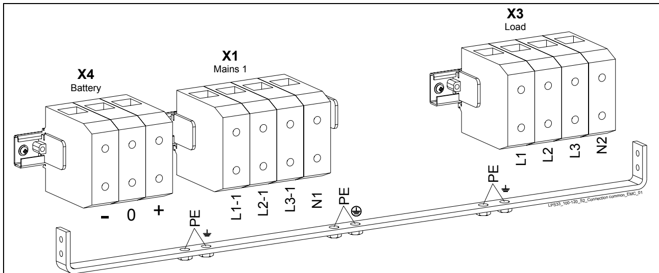
Рис. 5.8.3-1 Клеммы общего входа для подключения к электросети
