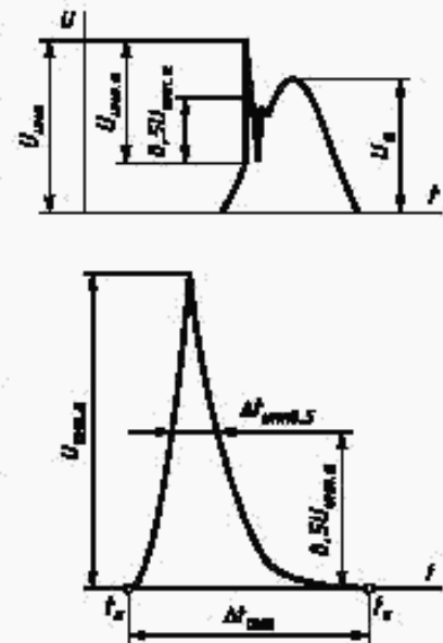
Рисунок Б.3 — Параметры импульсного напряжения
