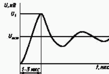
Рисунок Д.2 — Форма грозовых импульсов, характерная для точек присоединения а, в, з, д на рисунке Д.1.
