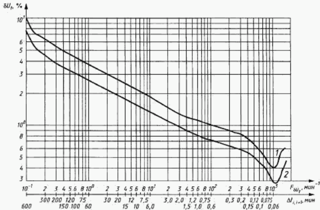
Рисунок 1 — Предельно допустимые размахи изменений напряжения в зависимости от частоты повторения изменений напряжения за минуту для колебаний напряжения, имеющих форму меандра
