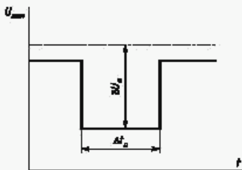
Рисунок Б.2 — Провал напряжения
