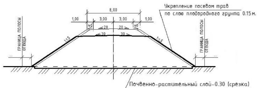
Тип 3 (насыпь до 6 м)
