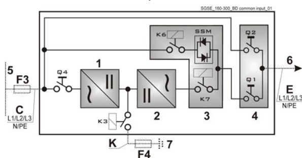
Общие входы выпрямителя и байпаса
